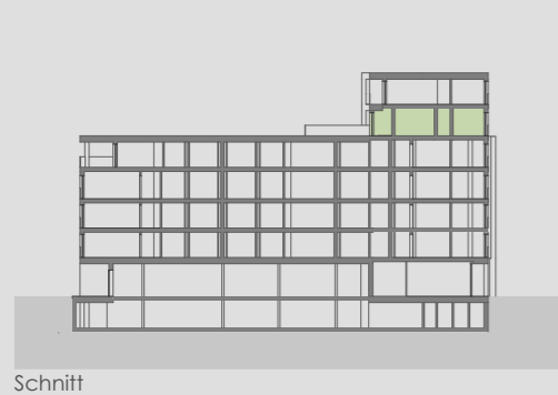
Schnitt
